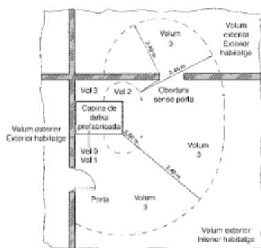
Figura 7 – CABINA DE DUTXA PREFABRICADA
